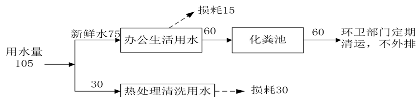
图 2-2 该期项目水平衡图 ( \text{m}^3/\text{a} )
