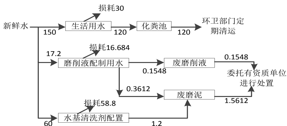
图 2-2 该项目水平衡示意图 ( \text{m}^3/\text{a} )
